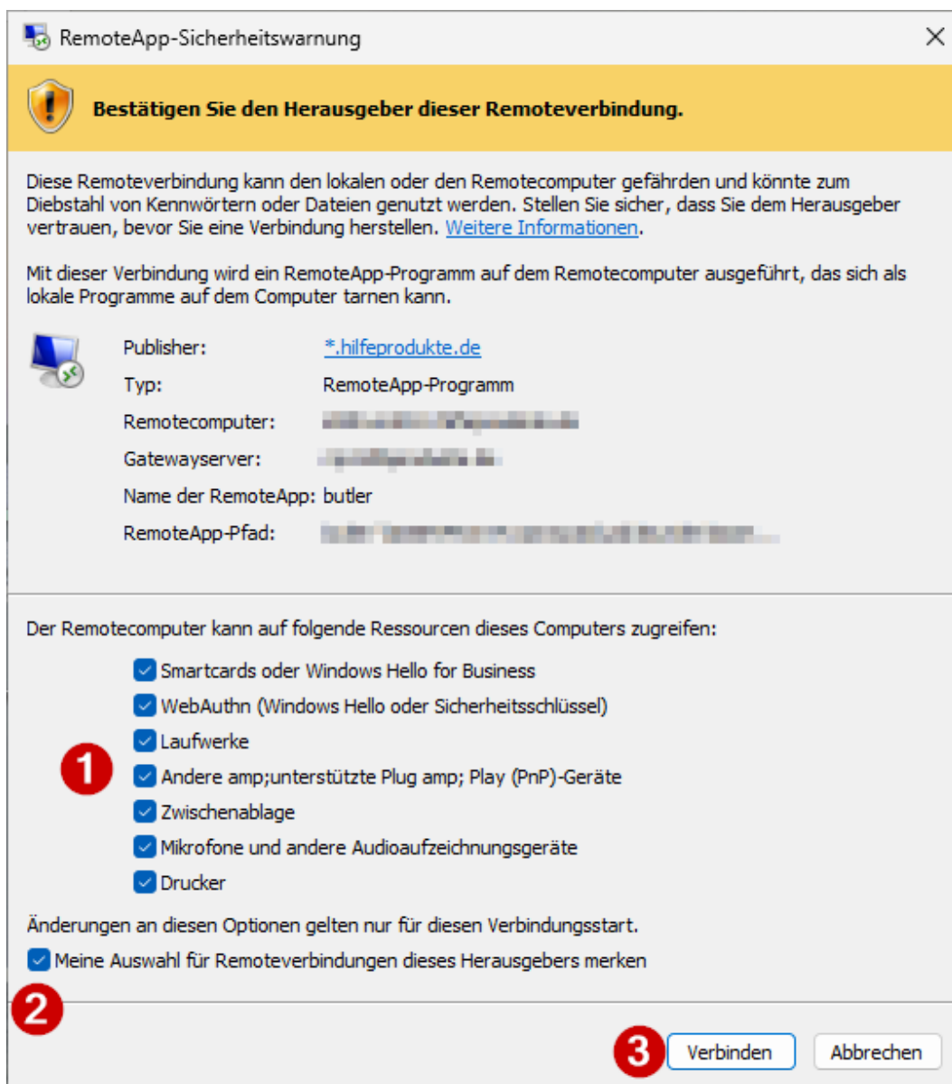
Bild 1: RemoteApp-Sicherheitswarnung
